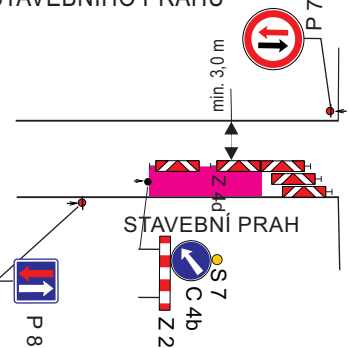
DETAIL - PRACOVNÍ MÍSTO PŘI VÝSTAVBĚ STAVEBNÍHO PRAHU
