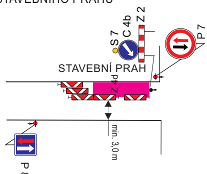
DETAIL - PRACOVNÍ MÍSTO PŘI VÝSTAVBĚ STAVEBNÍHO PRAHU
