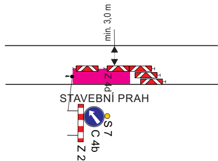
DETAIL - PRACOVNÍ MÍSTO PŘI VÝSTAVBĚ STAVEBNÍHO PRAHU
