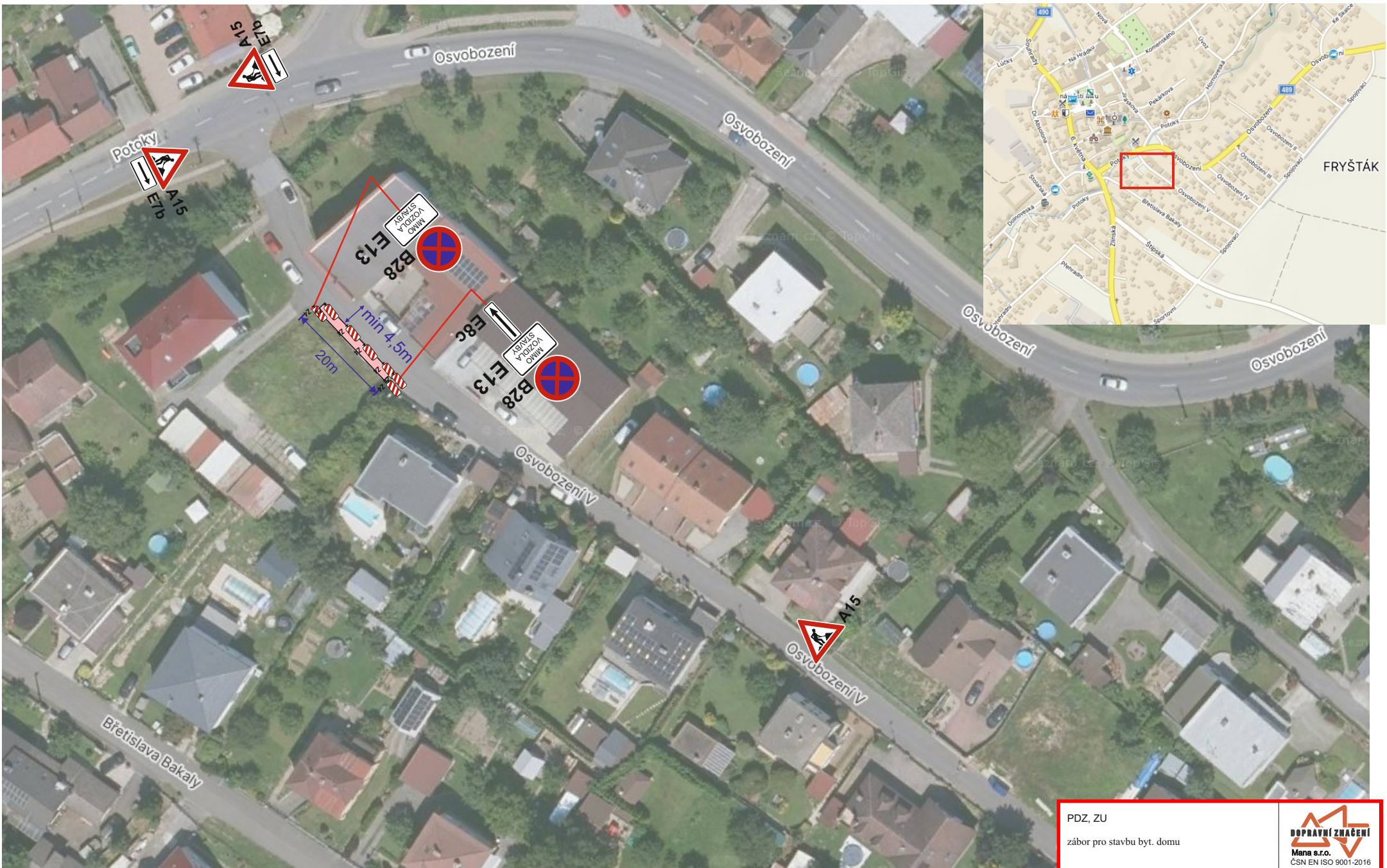
zábor pro vozidla stavby, zařízení staveniště
